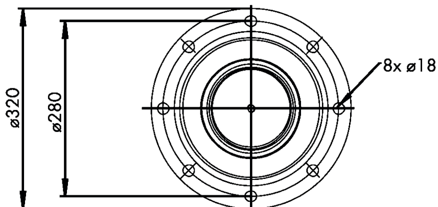
Hohlstrahldüse HS 130/10 E
