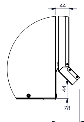
Dachrinne
