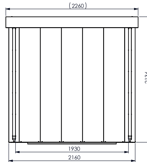
Von Hinten
