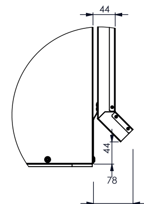
Dachrinne
