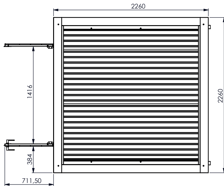
Von Oben
