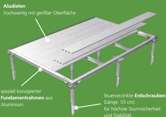
Abb. Erdschrauben-Fundament Gerätehaus HighLine Grösse H2
