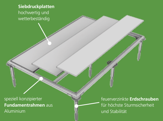
Abb. Erdschrauben-Fundament Gerätehaus HighLine Größe H2
